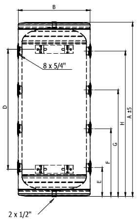
Crtež 2. za 80 i 100 litara sa osam bočnih priključaka
