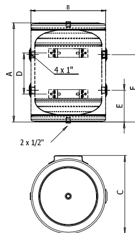
Crtež 1. za 30 i 50 litara sa četiri bočna priključka
